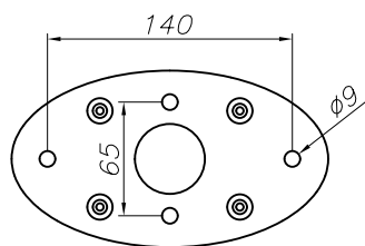
PLANTILLA DE INSTALACIÓN INSTALLATION TEMPLATE
