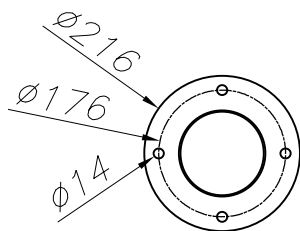
PLANTILLA DE INSTALACIÓN INSTALLATION TEMPLATE
